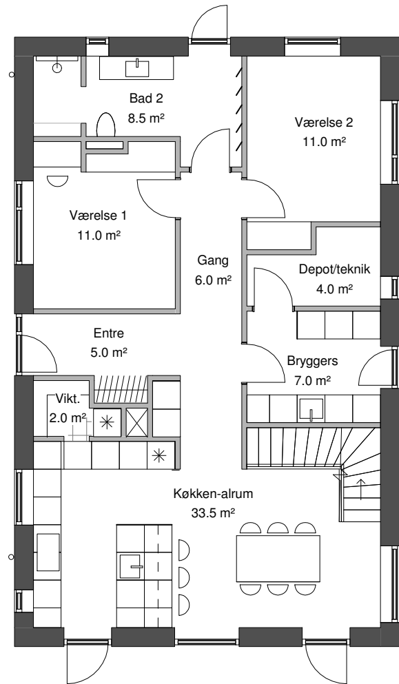
BOLIG - STUEPLAN
